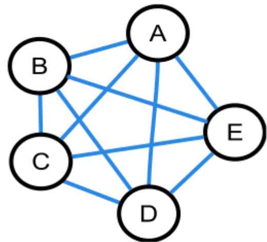
vollständiger Graph mit 5 Knoten
